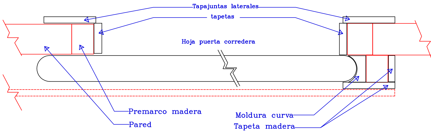
Esquema cierre puerta corredera interior pared
